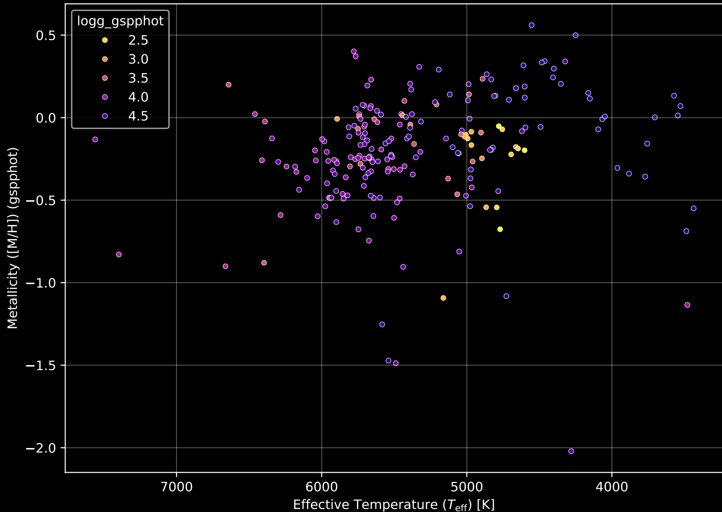
APOGEE DR17 Field: [251-33] Stellar Population Parameters (n= 214)
